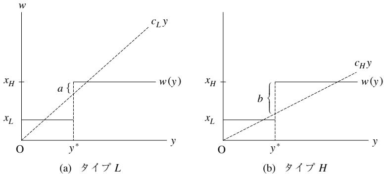
図2：分離均衡
